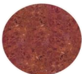
Яшма
