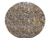
Гравий пёстрый
