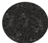
Габбро
